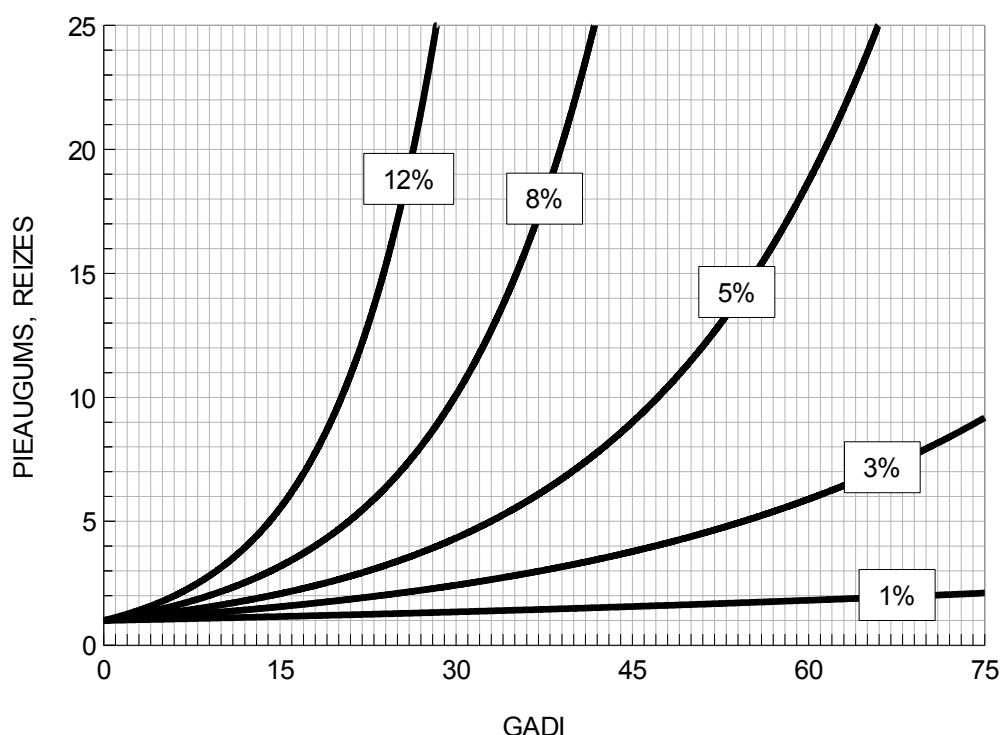
2. att. Eksponenciāla pieauguma līknes
